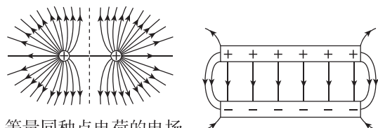
等量同种点电荷的电场 (负点电荷则方向相反) 匀强电场
