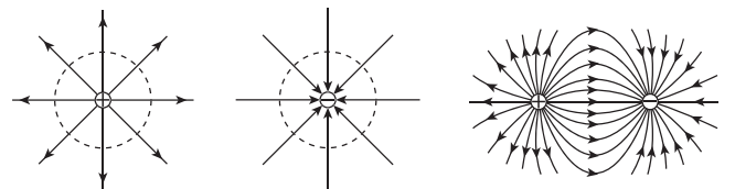
正点电荷的电场 负点电荷的电场 等量异种点电荷的电场
